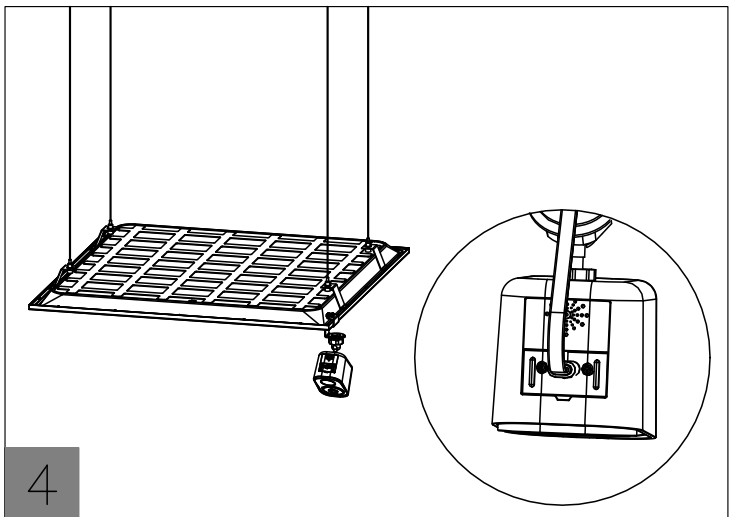
图片4：打开摄像头上的硅胶塞，将监控的电源Type-C线插入摄像头内。
