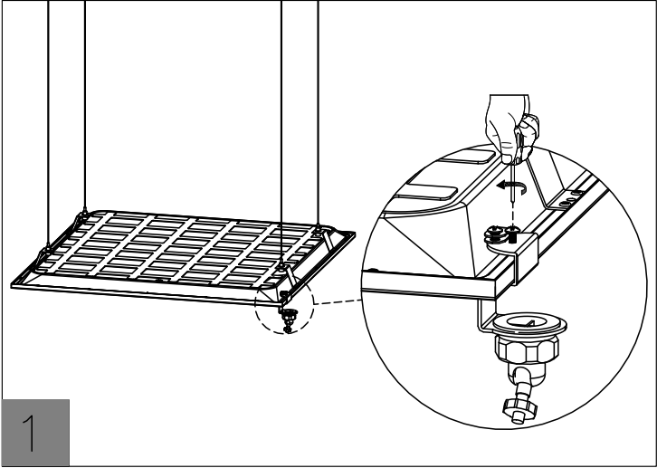
图片1：将监控支架套在面板灯的边框上，再锁紧支架上的螺丝。
