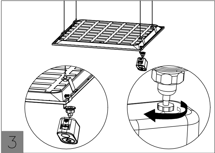
图片3：将摄像头锁在安装支架上，拧紧螺母。
