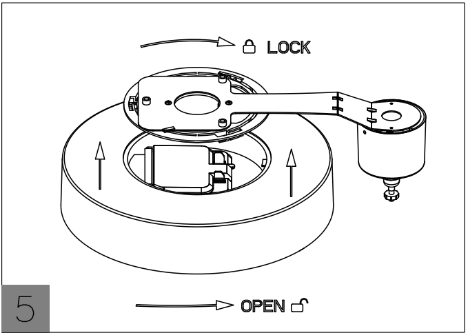
图片5：将灯具与安装底座对齐向上，然后旋转固定。
