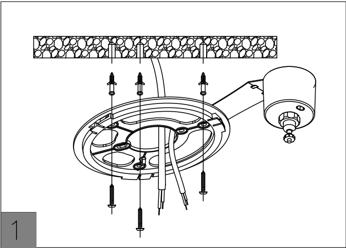
图片1：关闭电源，用膨胀螺丝将支架固定在天花板上。
