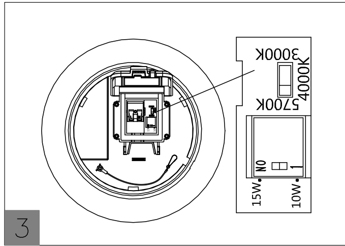
图片3：通过DIP开关选择所需的CCT和功率。
