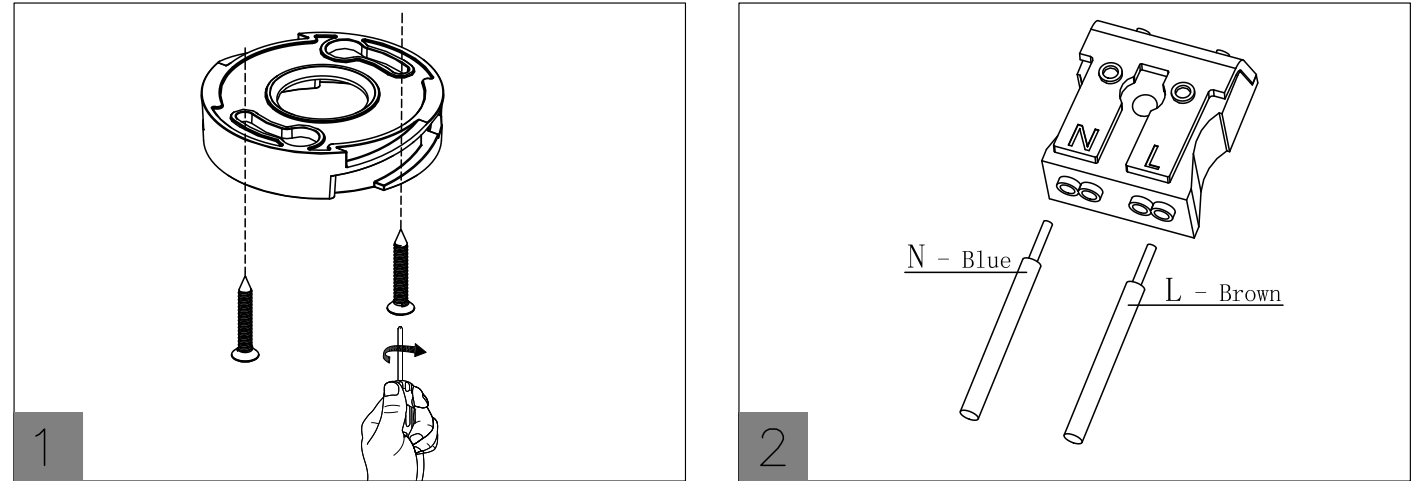
图片1：将底板固定在天花板上。
