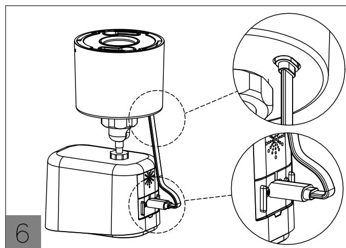
图片6：打开摄像头上的硅胶塞，将监控的电源Type-C线插入摄像头内。
