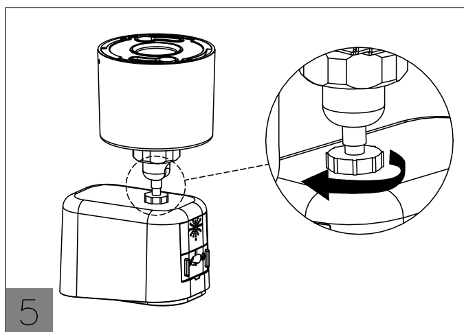
图片5：将摄像头锁在安装支架上，拧紧螺母。
