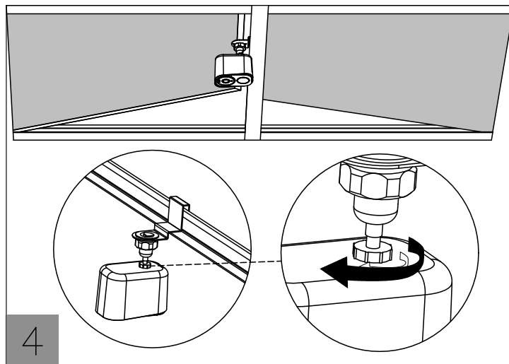
图片4：安装摄像头主体
