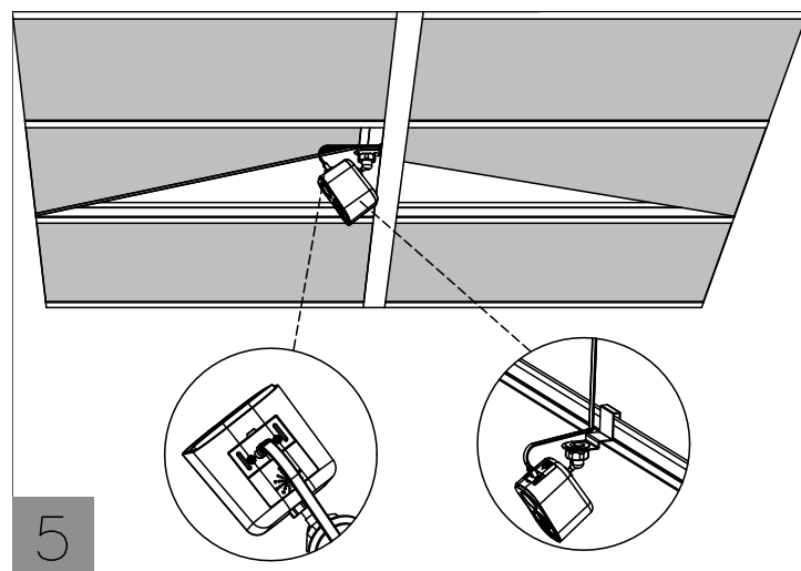
图片5：连接摄像头电源
