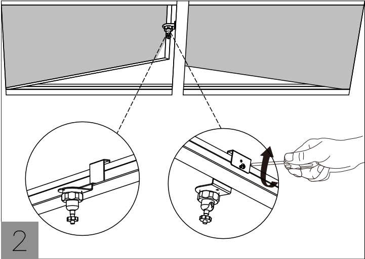
图片2：固定安装支架 将支架悬挂于龙骨上，拧紧支架侧面的固定螺丝。
