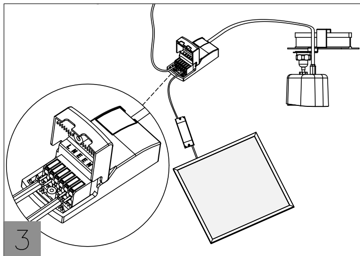
图片3：连接电源线路
